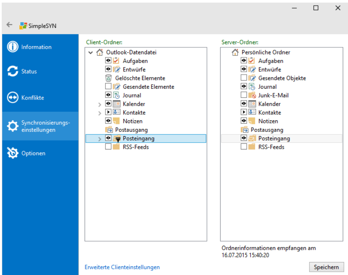
Abbildung 47: Ordner mit zugewiesenem Filter
