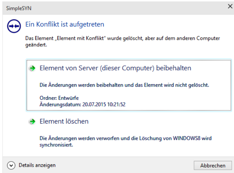
Abbildung 23: Dialog zur Konfliktlösung
